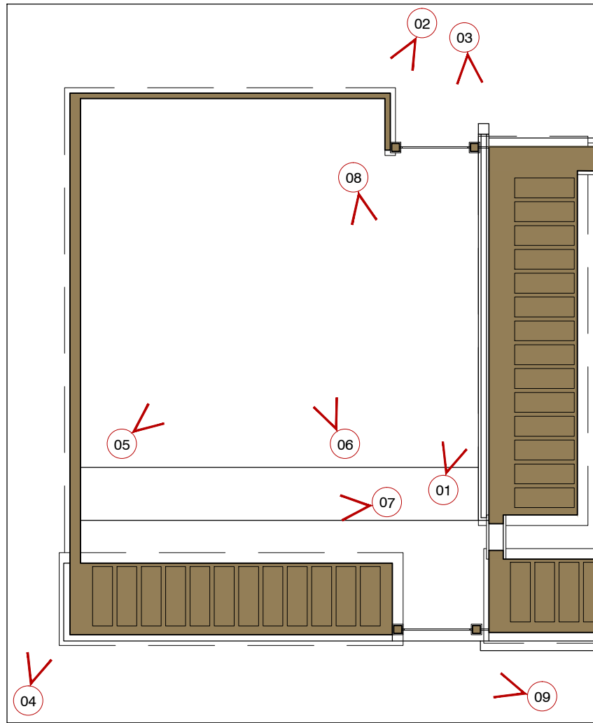
PLANIMETRIA CON INDICAZIONE DEI CONI OTTICI
